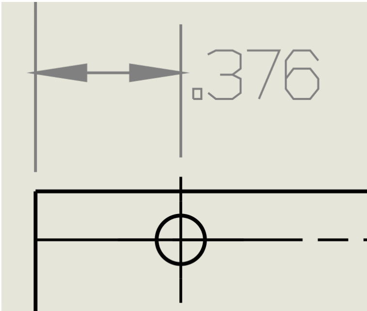
Rasterización activada
