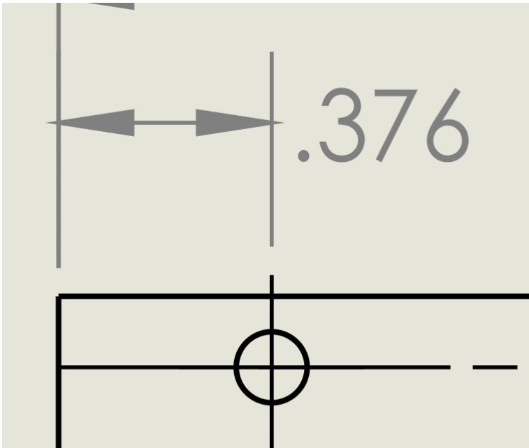
Rasterización activada
